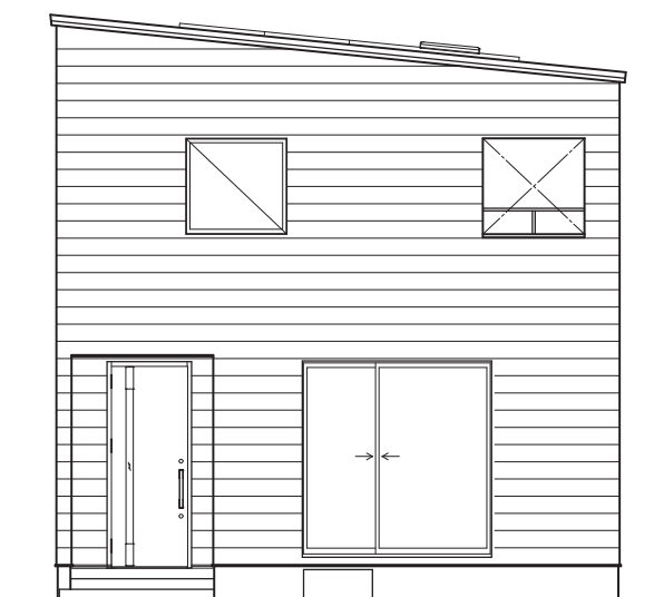
西側立面図
